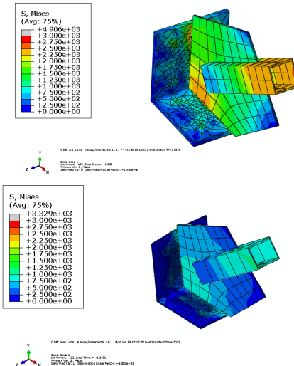
شکل ۳- توزیع تنش در اجزای اتصال در روش اتصال با پیچ و مهره
